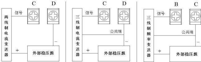
变送器接线方式 (外接稳压源)
