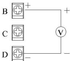
直流电压输入
